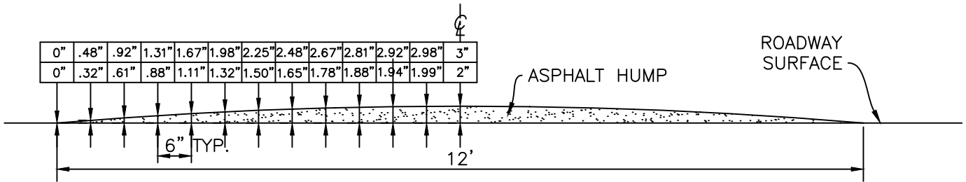
SECTION B-B SCALE: 1" = 2'
