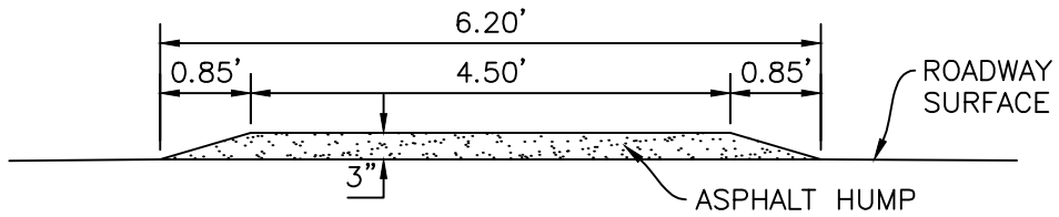
SECTION A-A SCALE: 1" = 2'
