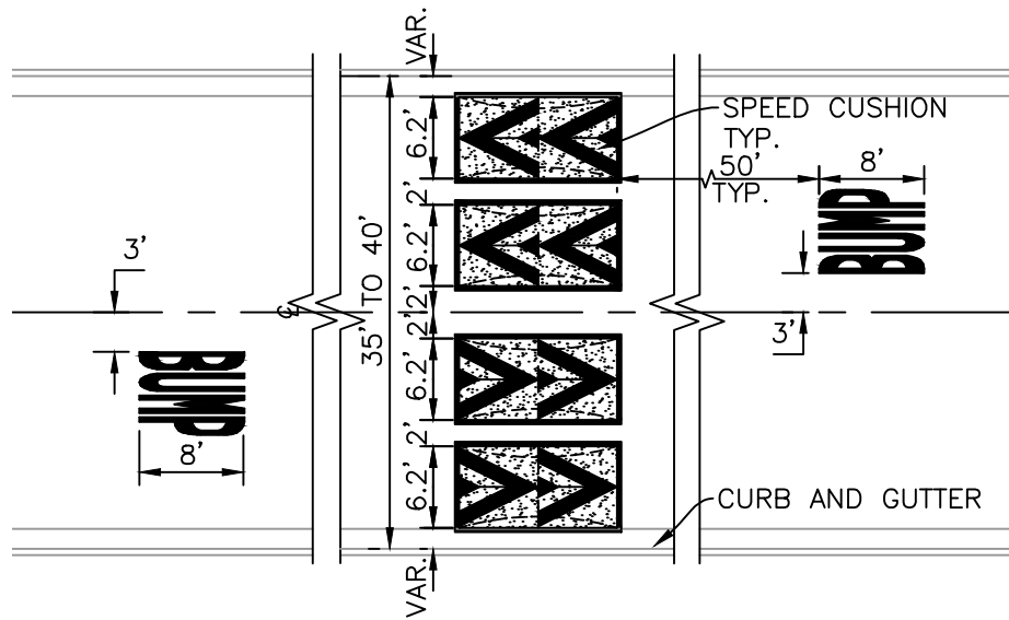
TYPE A SCALE: 1" = 16'
