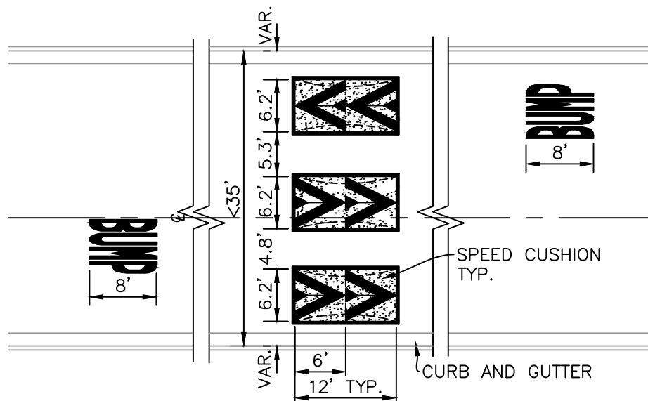
TYPE B SCALE: 1" = 16'
